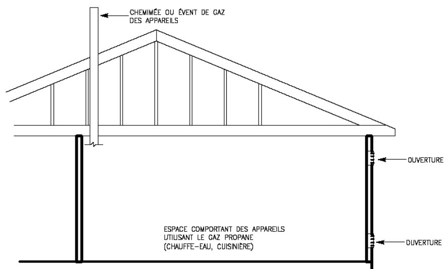
Figure 1.12.10.a - Exemple d'ouvertures directes sur l'extérieur
