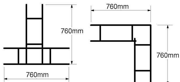
Té préfabriqué
