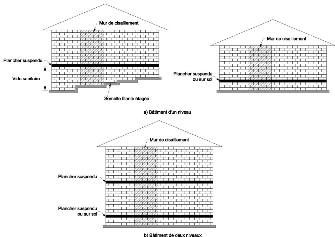
Figure 1.8.1 – Mur de cisaillement
