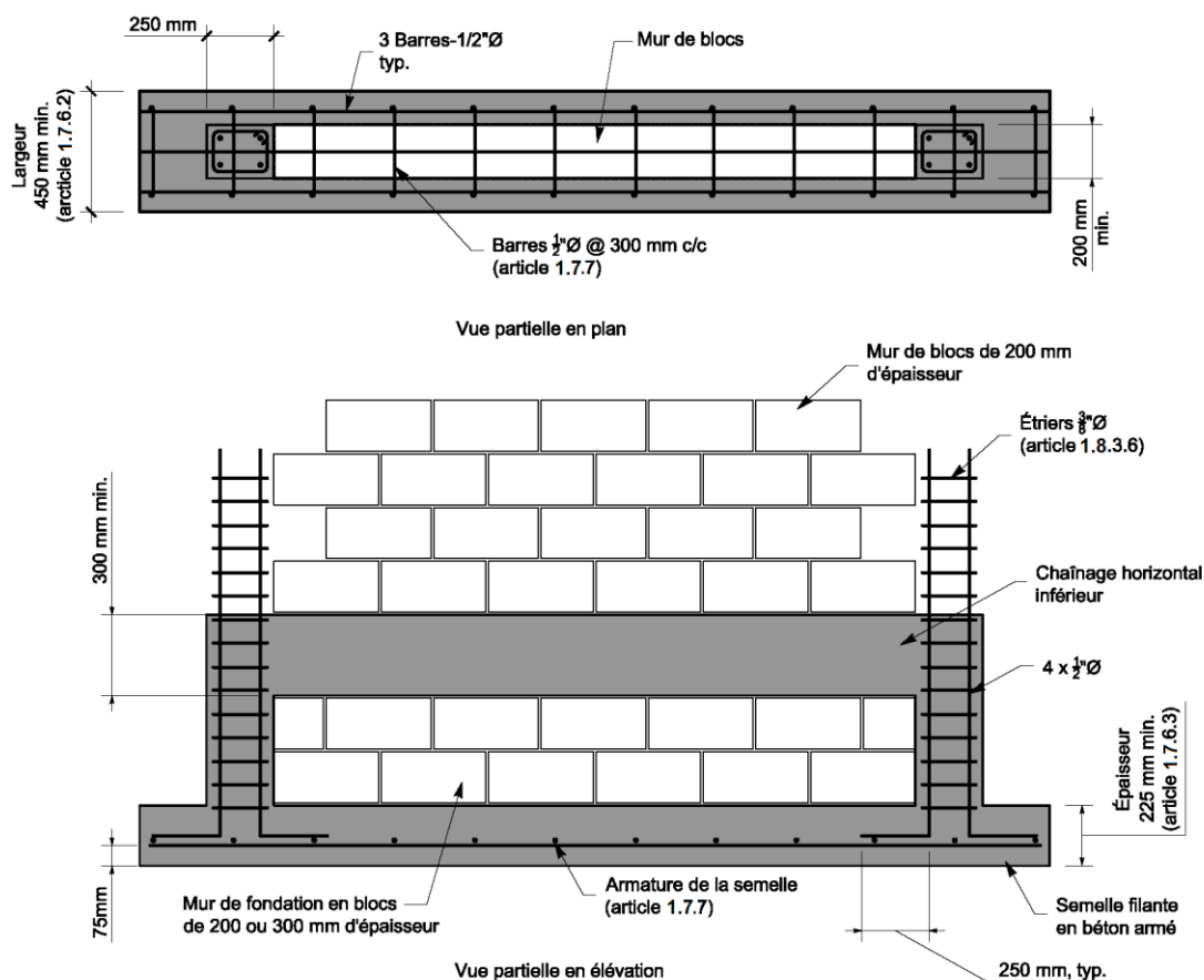
Figure 1.8.3.7 – Ancre des chaînages verticaux à la semelle de fondation
