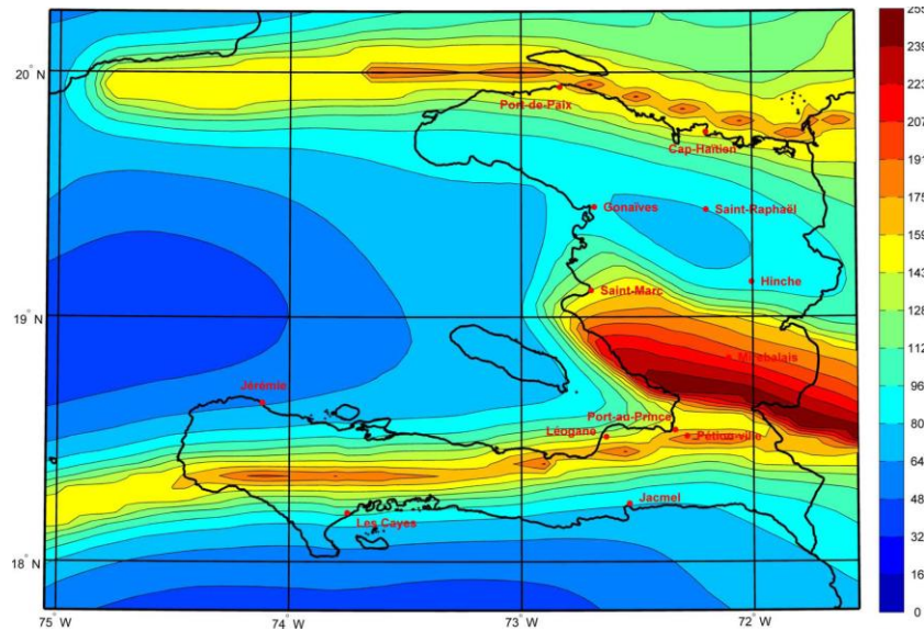
Figure 0.4.5.b – Spectre d'accélération pour une période de 0,2 s, pour 2 % de probabilité de dépassement dans 50 ans. Valeurs de dimensionnement (données USGS)
