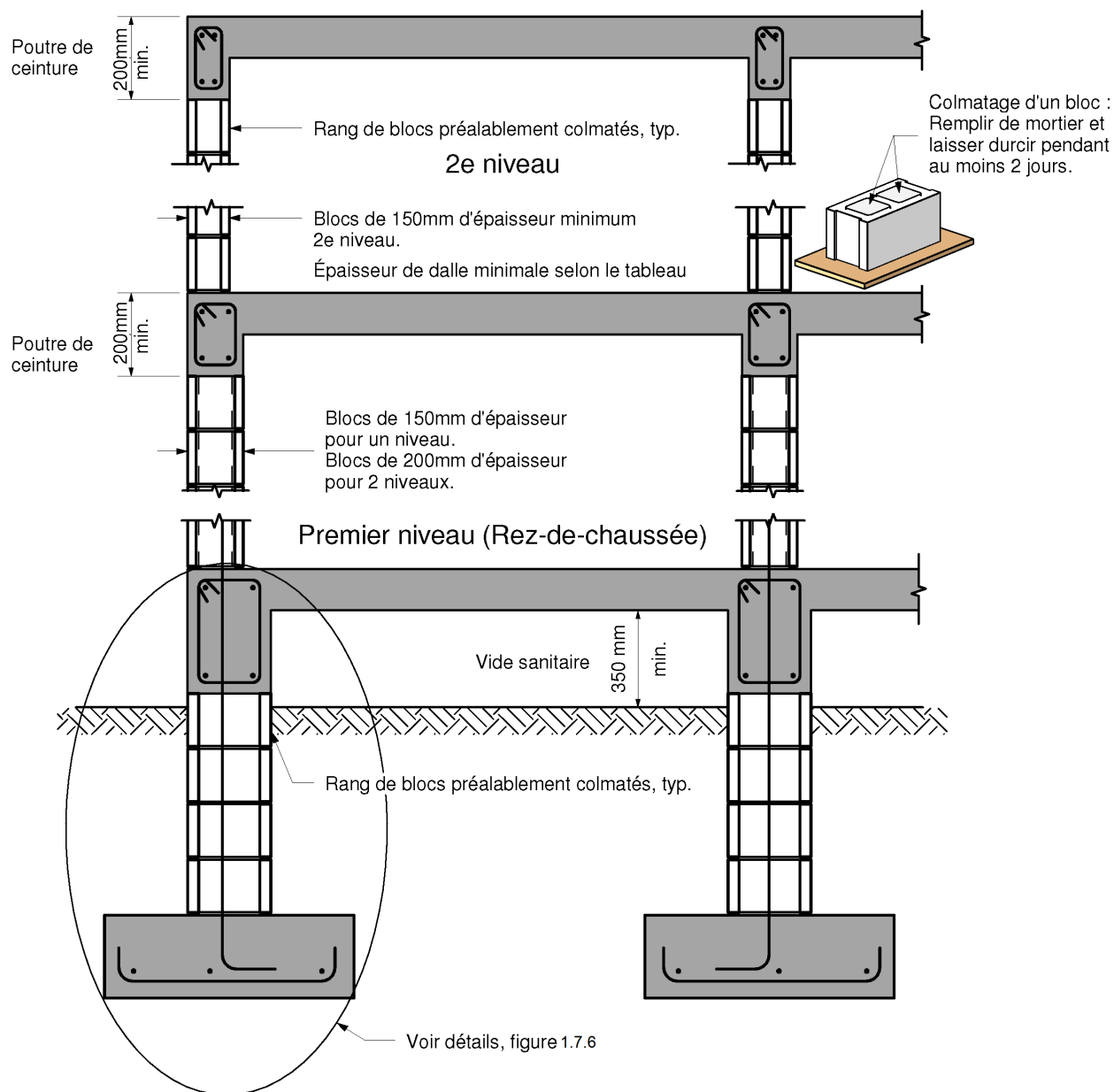
Figure 1.8.2.11.a - Emplacement des poutres de ceinture
