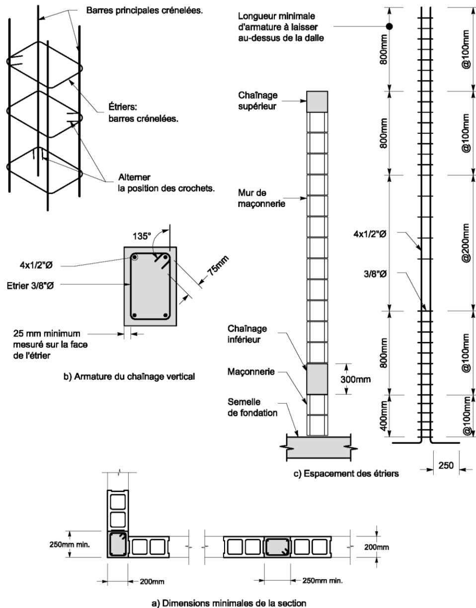
Figure 1.8.3.6 – Chaînages verticaux
