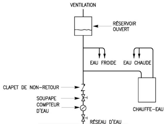
Figure 1.13.5.3 – Réservoir ouvert à la pression atmosphérique (schéma type)
