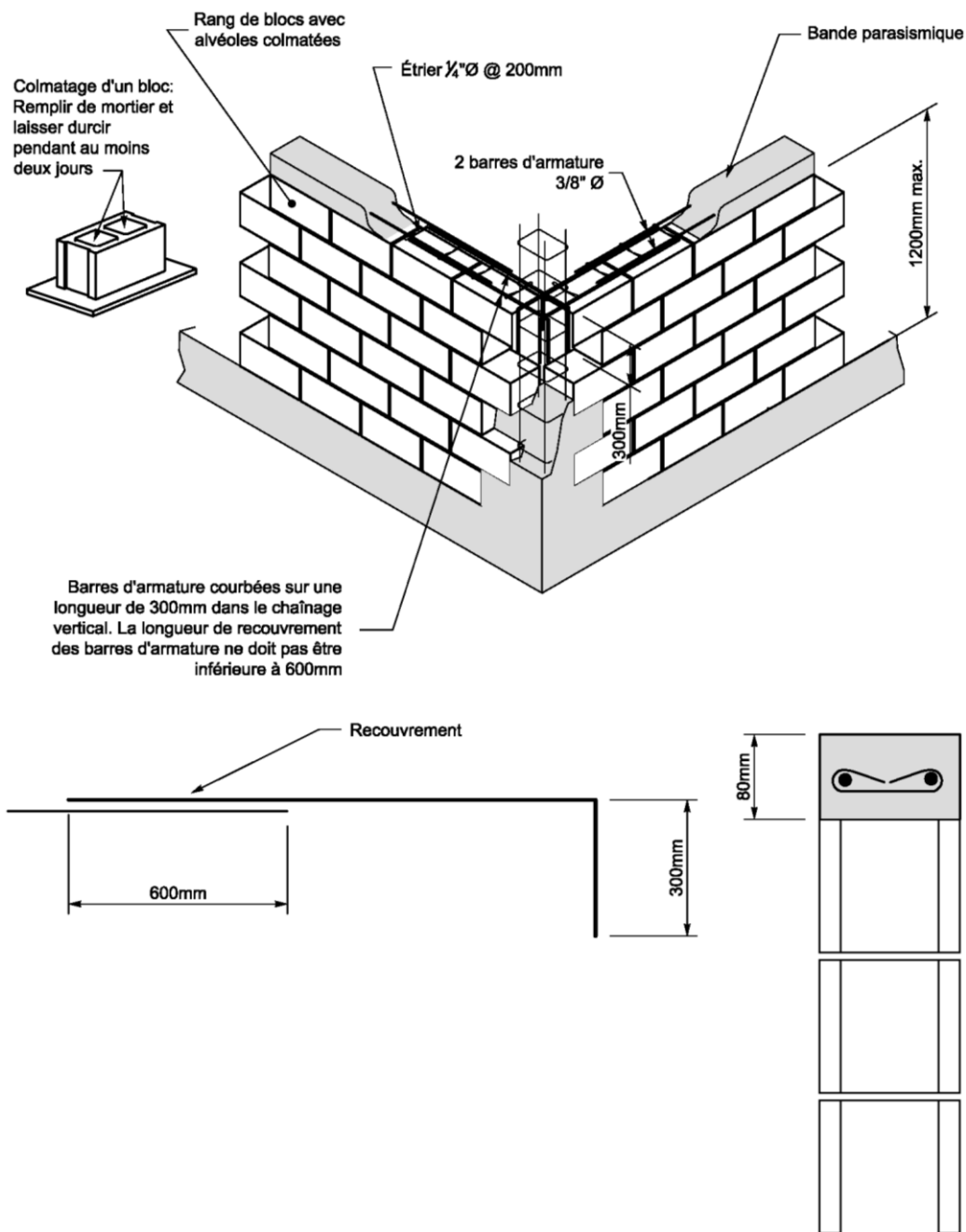
Figure 1.8.3.11.b - Bande parasismique
