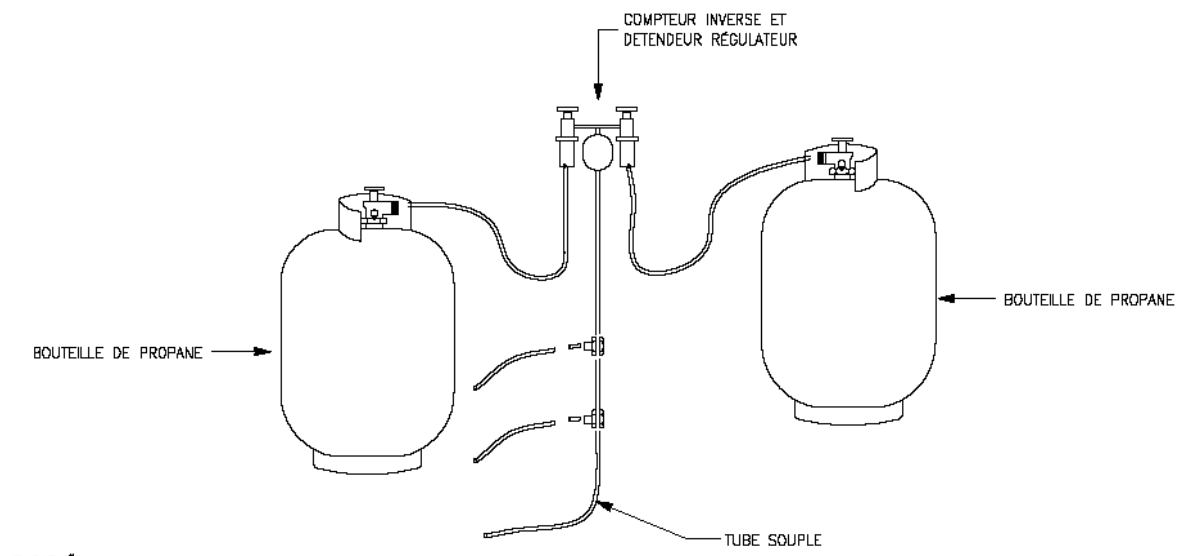
Figure 1.12.7.2.b - Bouteilles multiples
