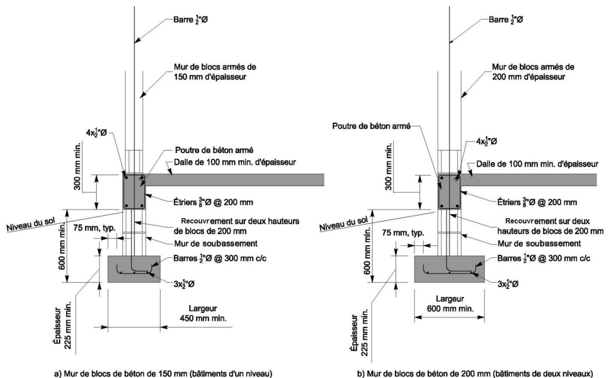
Figure 1.7.6.3 – Semelles filantes pour les murs de maçonnerie armée
